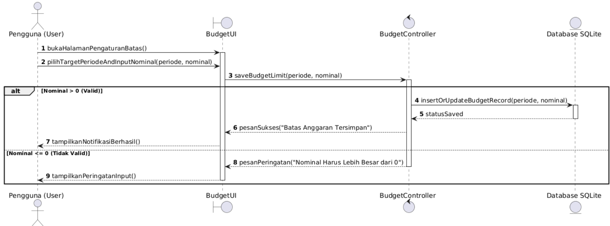
Sequence Diagram UC-09: Mengatur Batas Pengeluaran
