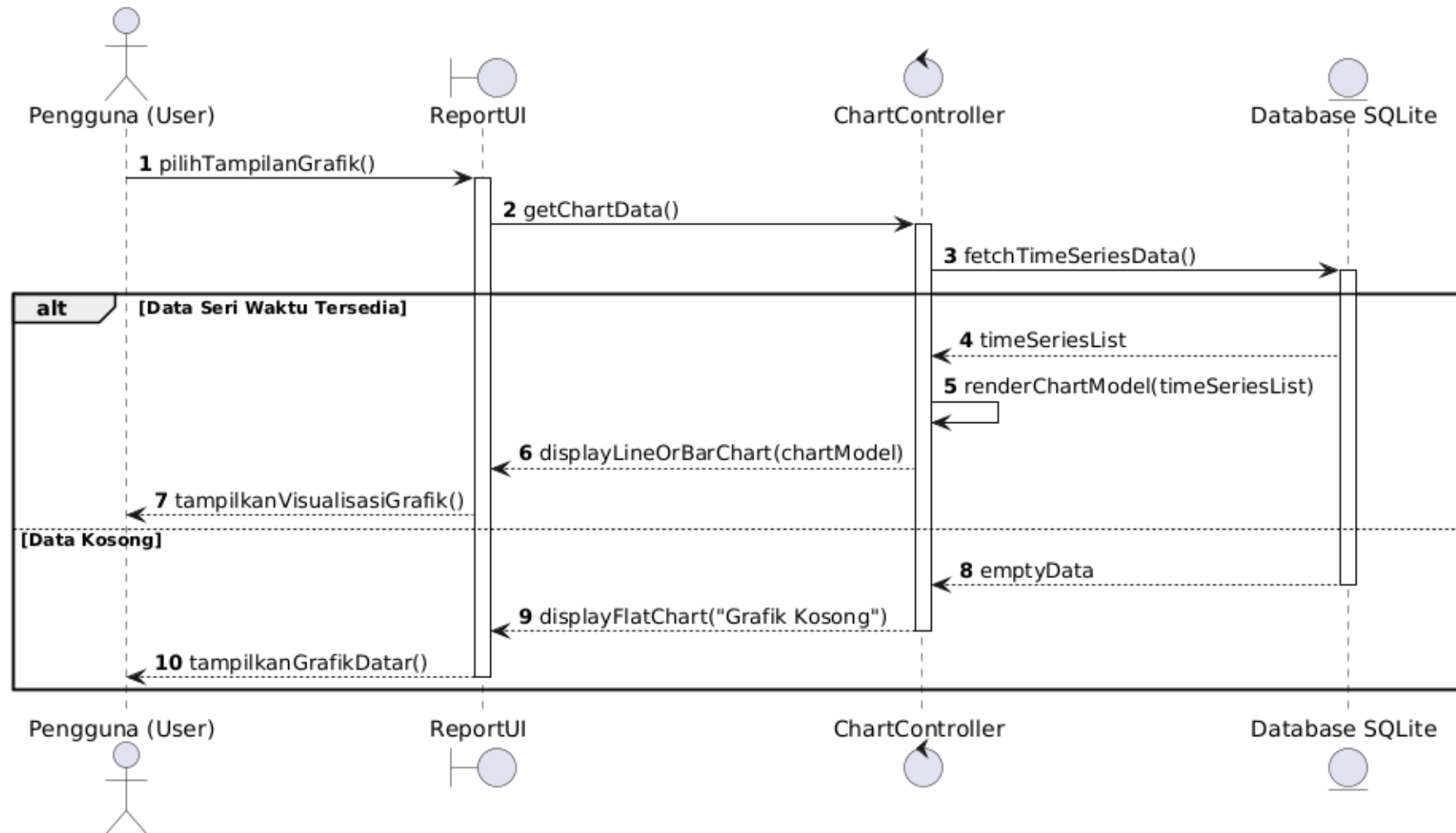
Sequence Diagram UC-13: Melihat Grafik Tren Keuangan
