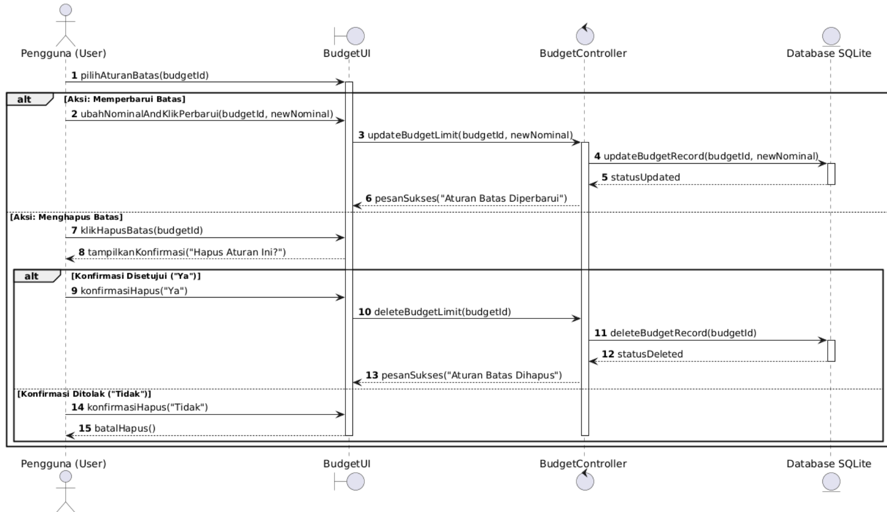
Sequence Diagram UC-10: Memperbarui atau Menghapus Batas
