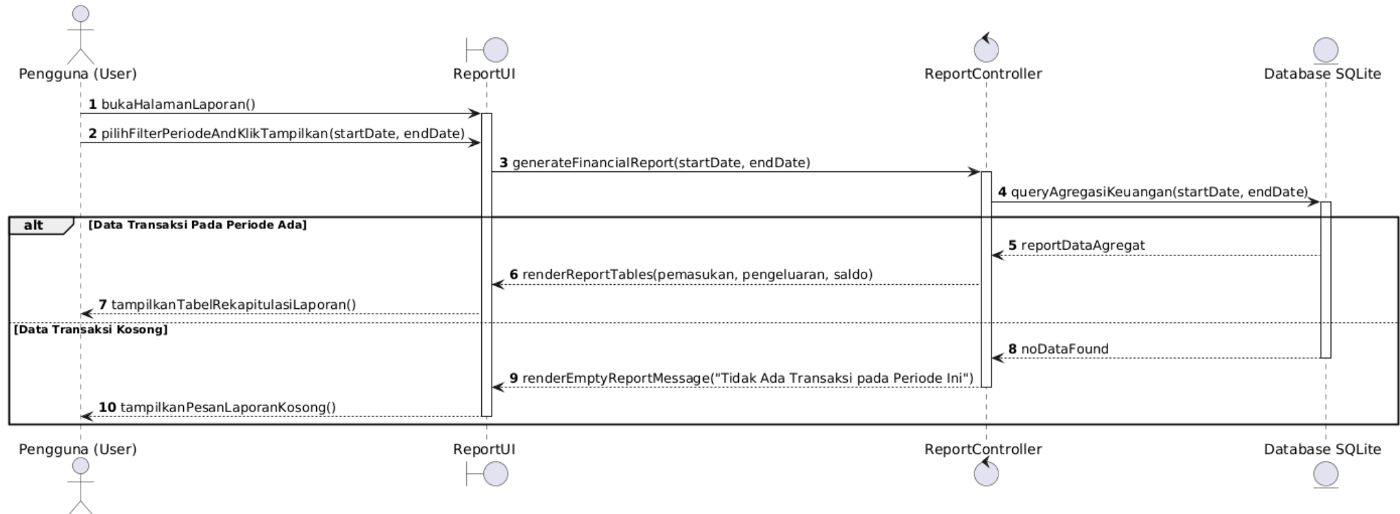
Sequence Diagram UC-12: Melihat Laporan Keuangan
