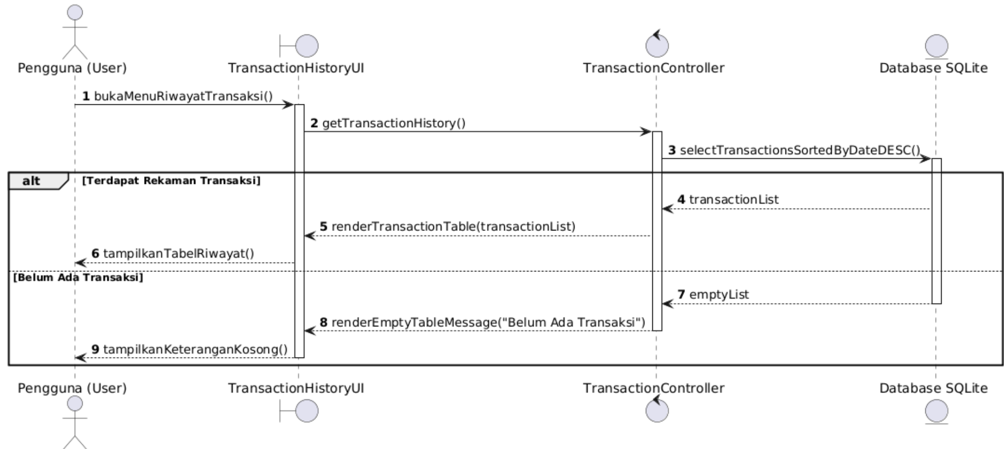
Sequence Diagram UC-03: Melihat Riwayat Transaksi
